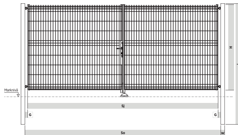
MODEST-port med dubbla blad sedd inifrån
