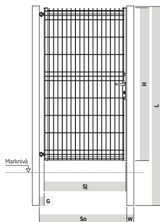
MODEST-grind sedd inifrån
